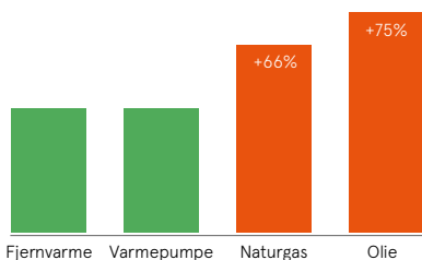
CO 2 -UDLEDNING*
